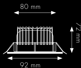
8 W Deckenausschnitt 85 mm
