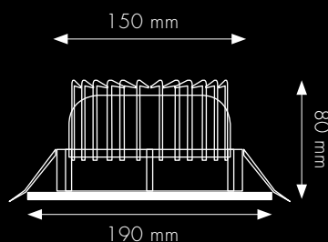
24 W / 32 W Deckenausschnitt 175 mm
