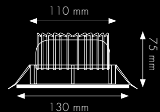
16 W Deckenausschnitt 118 mm
